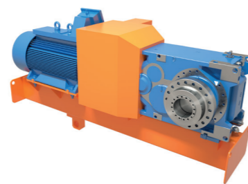
Vollwelle mit Flanschkupplung und Motorschwinge
