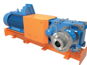
Vollwelle mit Abtriebskupplung und Motorrahmen
