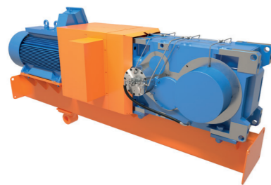
Arbre creux avec frette de serrage et châssis avec bras de réaction
