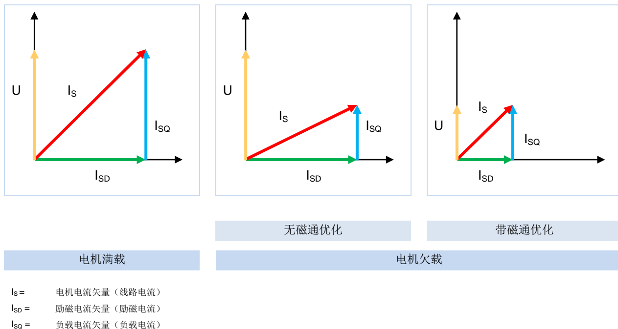
图 19: 自动励磁优化导致的能量效率
