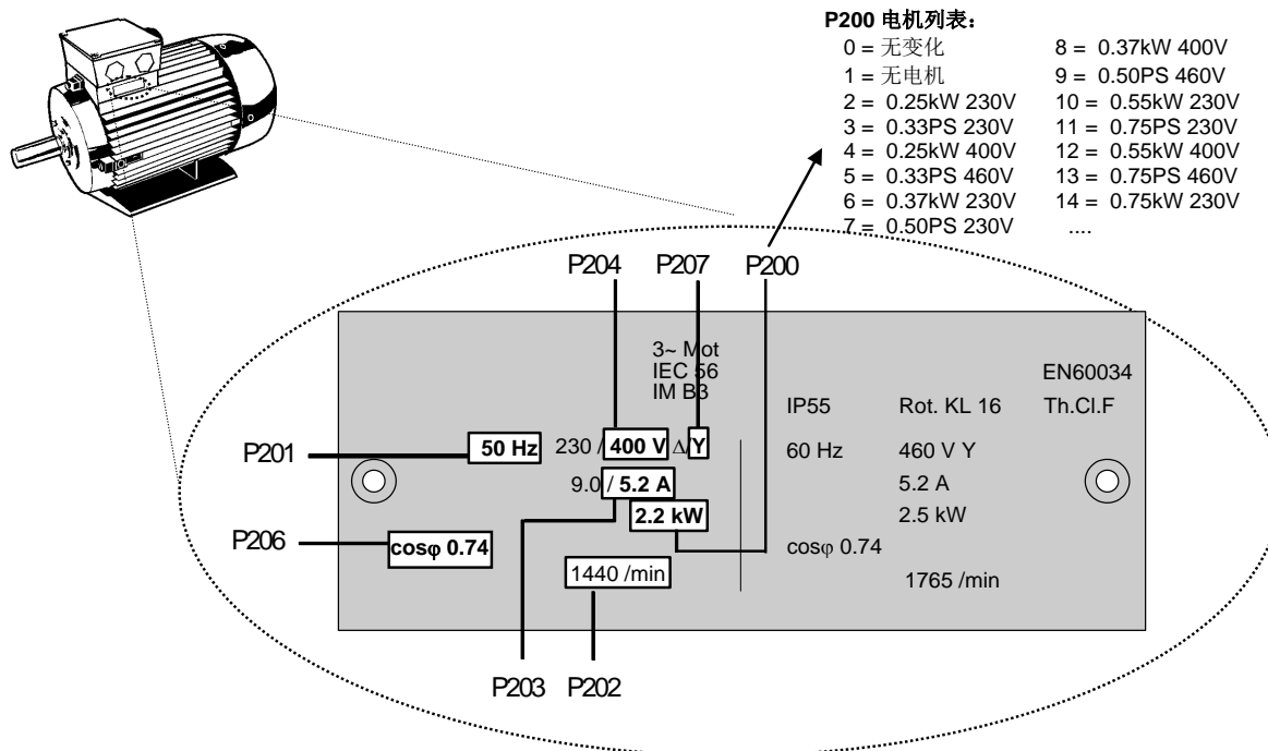
图 13: 电机铭牌
