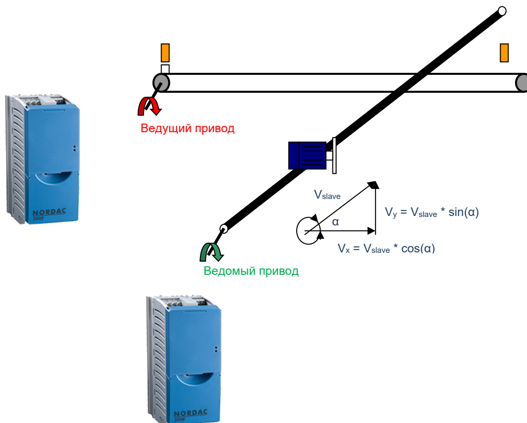
Рис. 5: Летающая пила, диагональная пила
