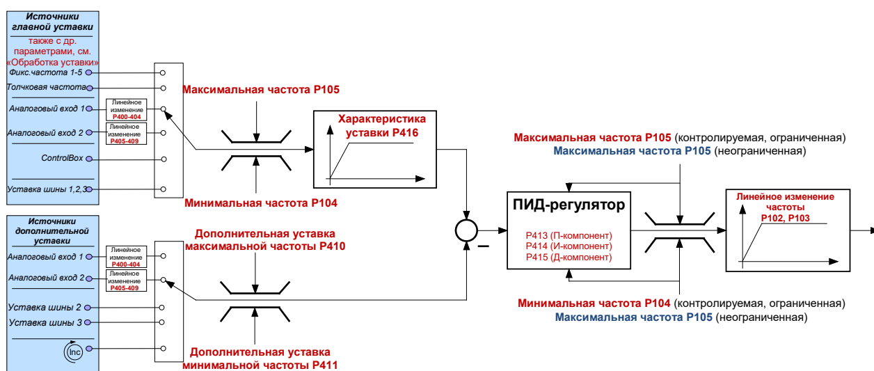
Рис.: Схема ПИД-регулятора
