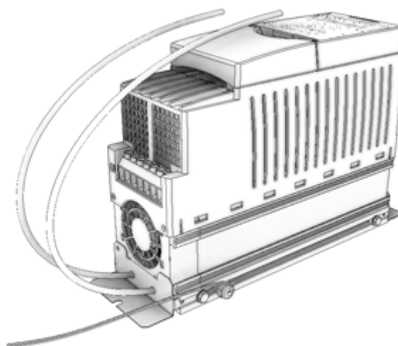
Пример: SK 500E типоразмера 2 и BR4-75-... с реле температуры (артикул 275991200)
