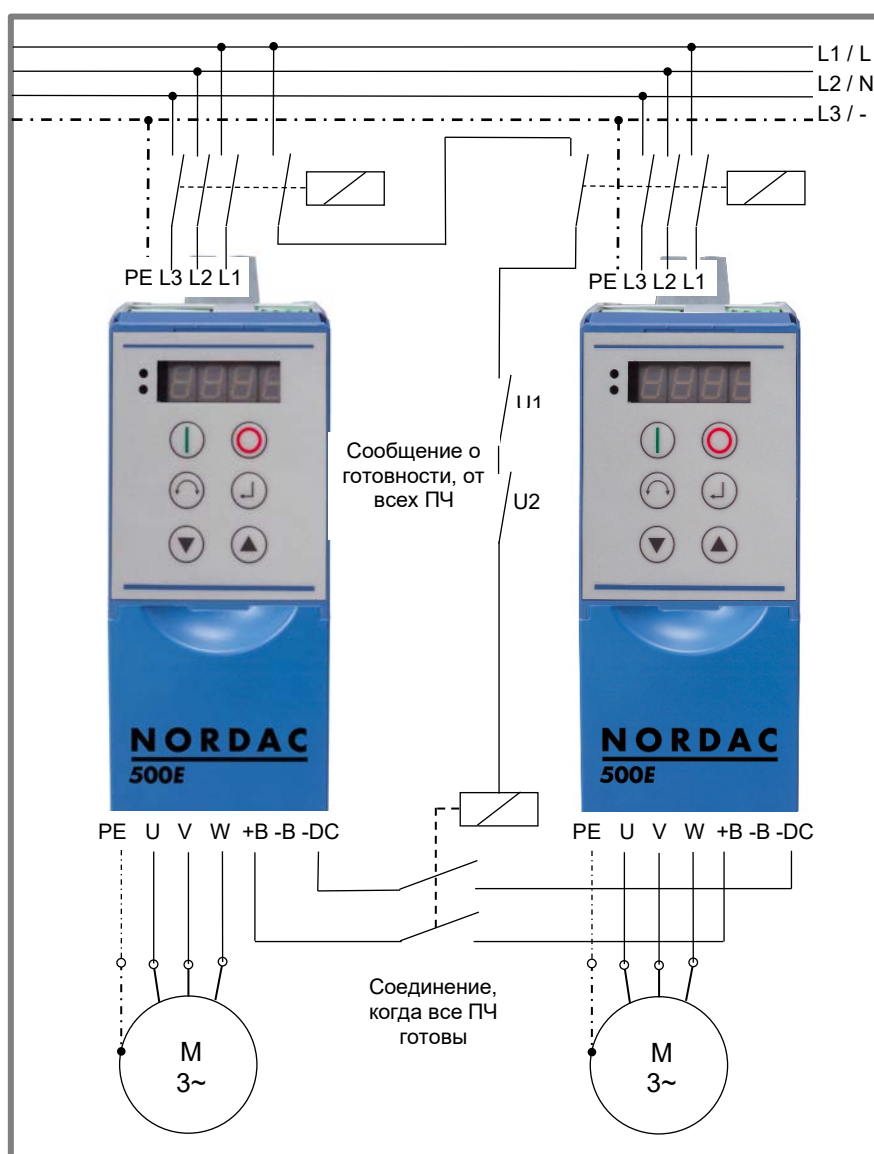
Рисунок 7: Схема прямого подключения к источнику постоянного напряжения
