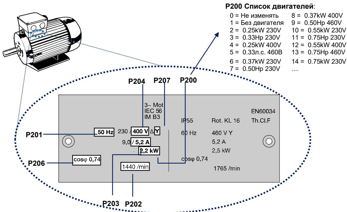
Рисунок 12: Заводская табличка двигателя
