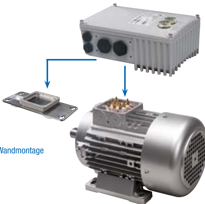
Motormontage
