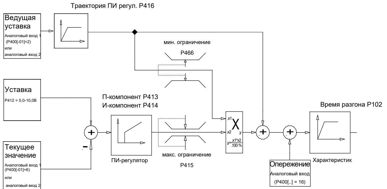
Рисунок 14: Блок-схема работы регулятора процесса
