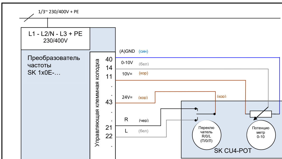
Рис. 11: Схема подключения SK CU4-POT, пример для SK 1x0E
