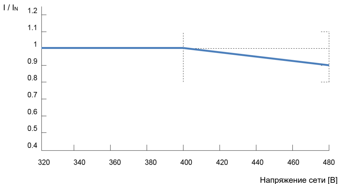
Рис. 18: Выходной ток в зависимости от сетевого напряжения
