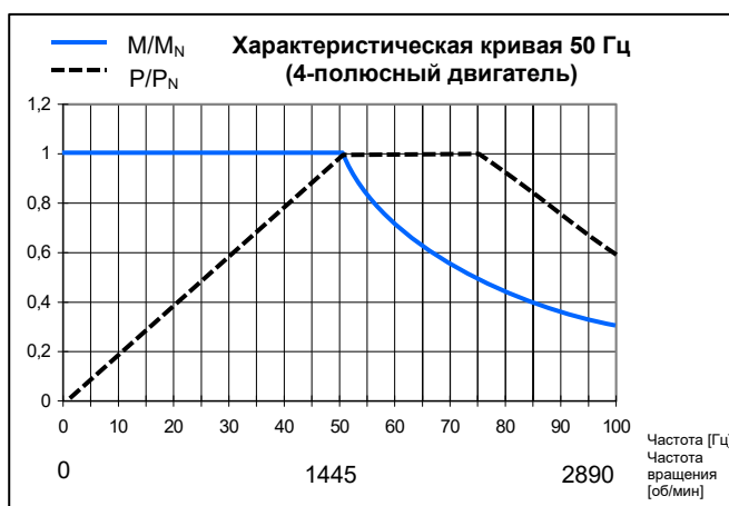
Рис. 20: Характеристическая кривая 50 Гц
