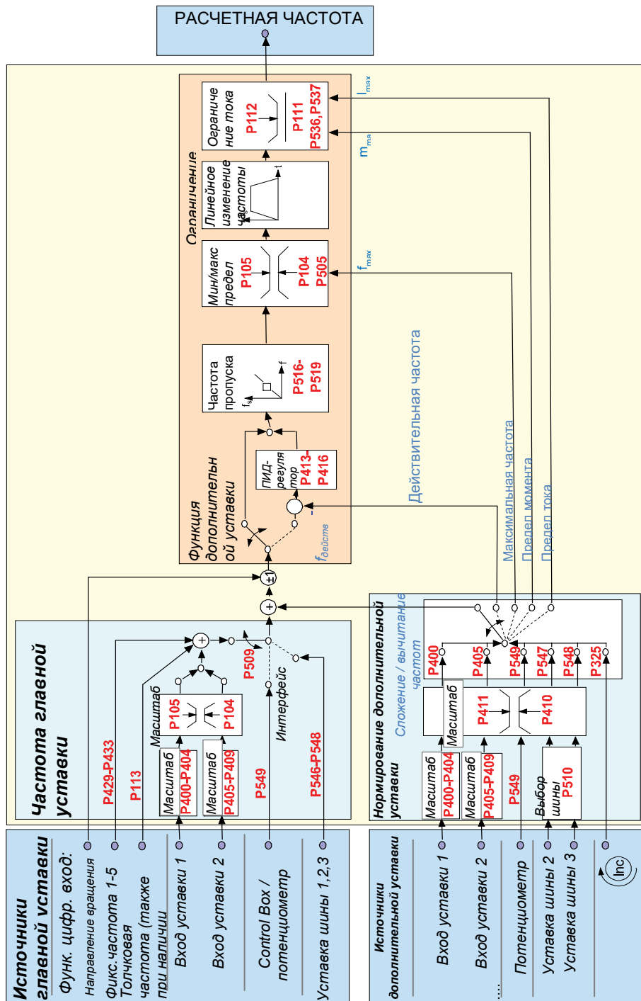
Рис. 13: Обработка уставки
