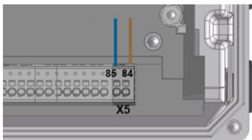
Рис. 12: Соединительные клеммы AS-i
