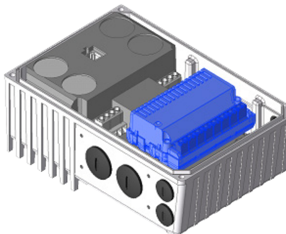
Рис. 1: Устройство со встроенным модулем SK CU4-...
