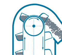
Élévateur à godets centrifuges
